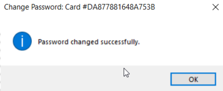
Εικόνα 26-Change token password
